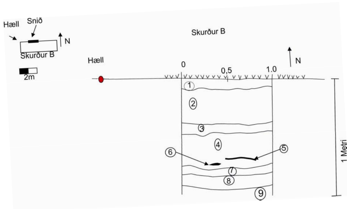
Teikning 2. Snið af skurði B. Teikning GJP, tölvuvinnsla MHH.
