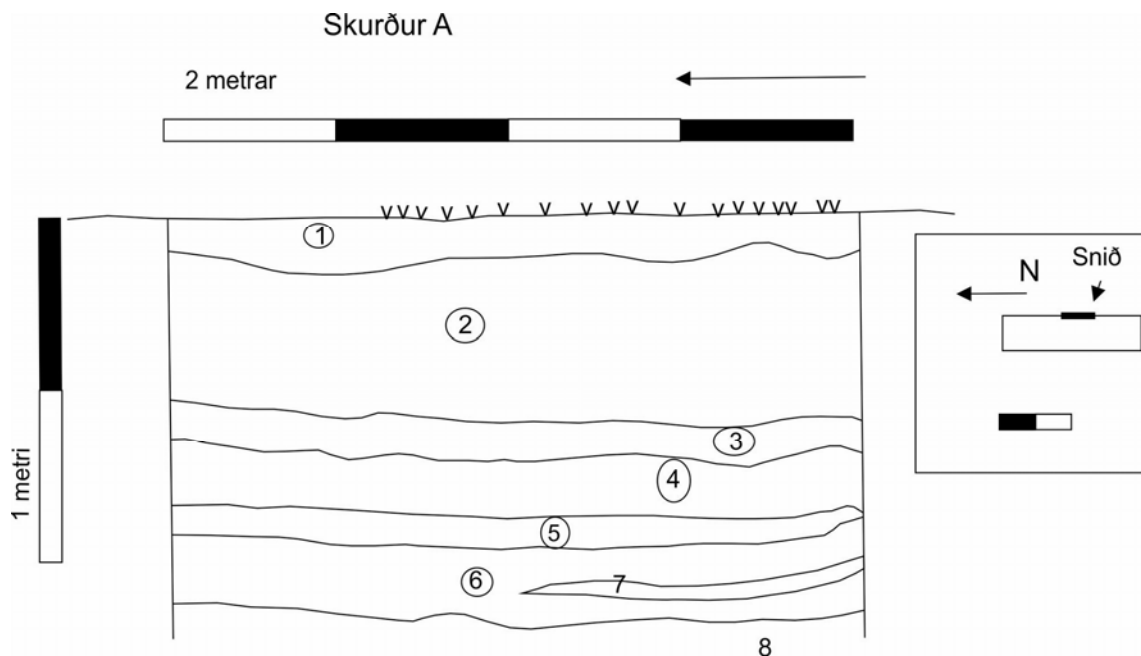
Teikning 1. Snið af skurði A. Teikning GJP. Tölvuvinnsla MHH.
