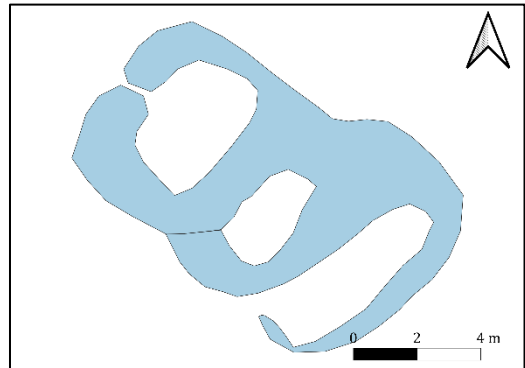
Mynd 22. Uppmæling af tóft 3121-011.
